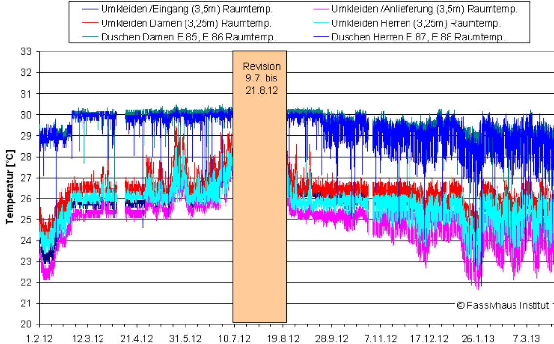
Abbildung 48: Verlauf der Raumlufttemperaturen vom Umkleidebereich und der Duschen vom 01.02.2012 bis zum 01.04.2013 (Stundendaten)
