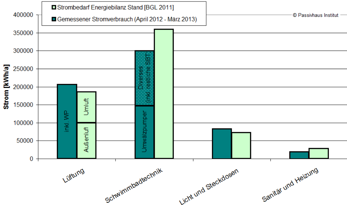
Abbildung 110: Gegenüberstellung des projizierten Strombedarfs während der Planungsphase mit den Messdaten aus dem Jahr April 2012 – März 2013 nach verschiedenen Teilbereichen.
